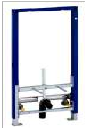
Duofix Bidet-UP-Element. Für die Montage vor eine tragende Wand. H = 112 B = 50 T = variabel. Auch in Bauhöhe 85 cm lieferbar.
