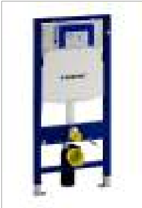
Duofix Spülkastenelement für die Montage vor eine tragende Wand. H = 112 B = 50 T = variabel. Mit Spülkasten Typ UP320, für alle Betätigungen der Sigma-Reihe.
